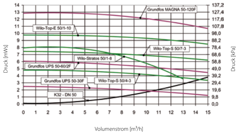
Differenzdruckdiagramm K32
