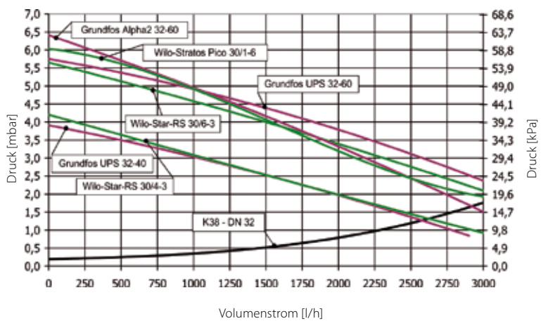
Differenzdruckdiagramm K38
