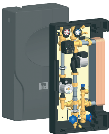
Módulo transmisor de calor para acumulador
