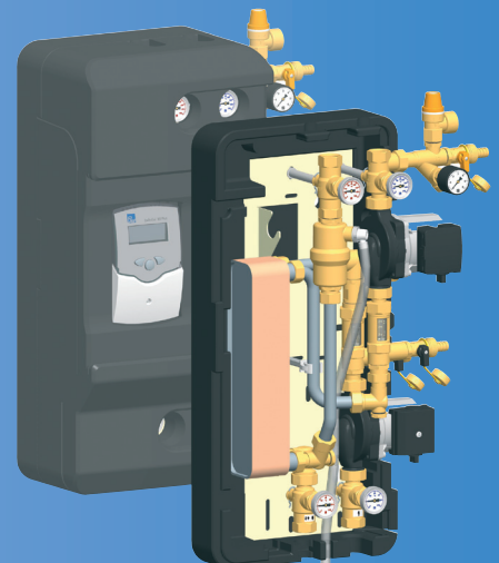
SolexMini
