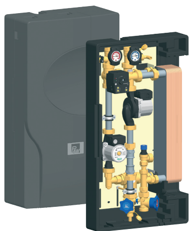
Stazione di trasferimento tra accumulatori
