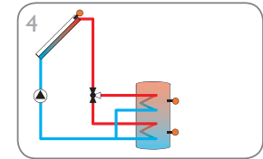
Solarsystem mit 1 Speicher und 3-Wege-Ventil zur Speicherschichtladung (Seite 11)
