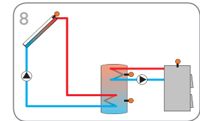
Solarsystem mit 1 Speicher und Festbrennstoffkessel (Seite 15)
