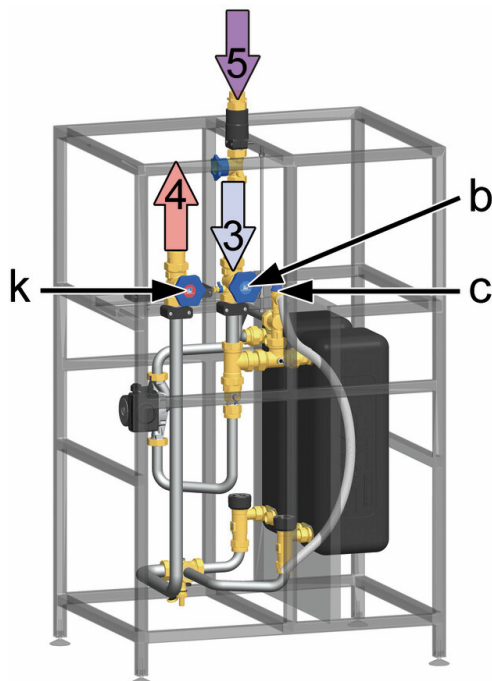
Circuito secondario
