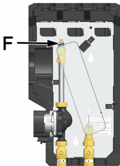
Circuit primaire
