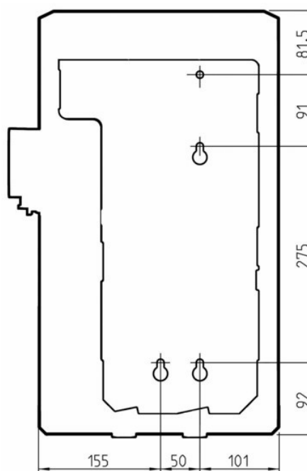
gabarit de perçage
