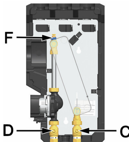
Circuit primaire
