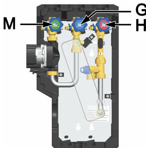
Circuit secondaire
