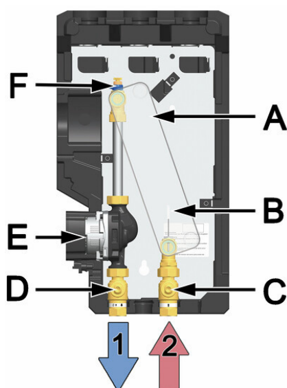
Circuit primaire
