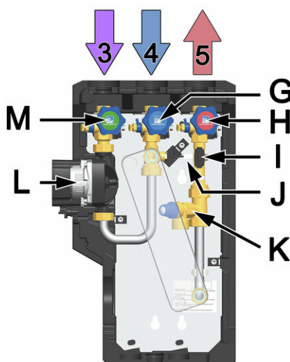
Circuit secondaire
