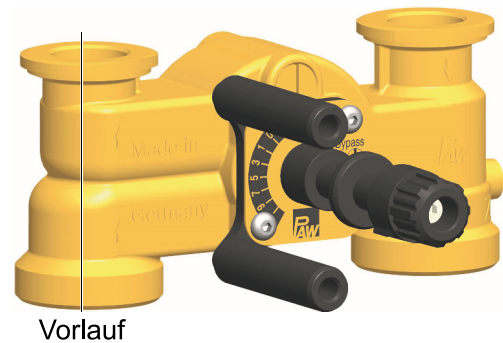
Mischer mit Vorlauf links
